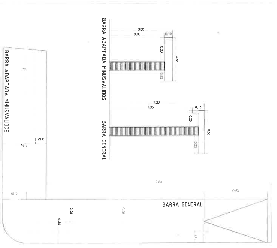
DETALLES BARRA
